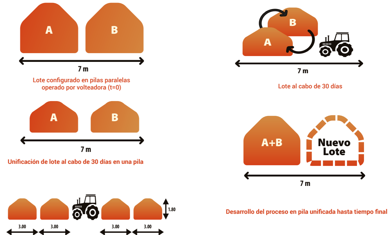
Figura 11. Detalle de pilas de compost.
