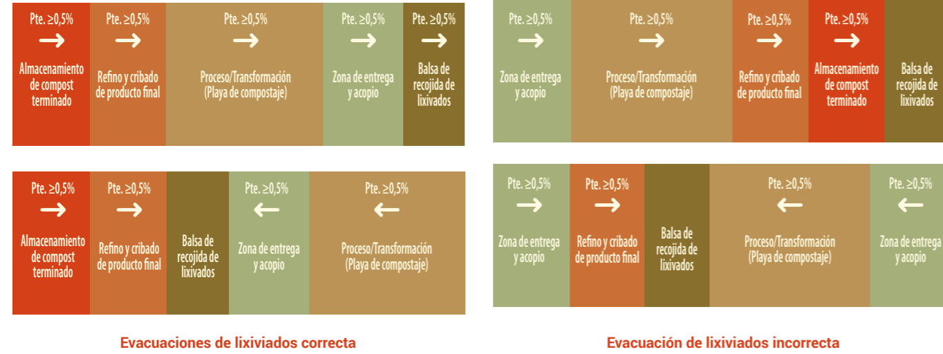
Figura 12. Recomendaciones de diseño para que el flujo de lixiviados discurra de forma adecuada (sin escala).
