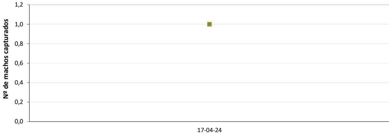
Nº de capturas de machos de Aonidiella aurantii : Vila-real (por día)
