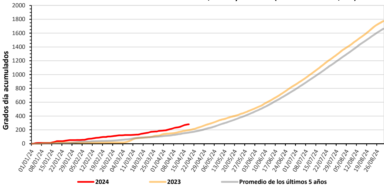
Grados día acumulados: Castelló Benadresa, Onda y Vila-real (valor umbral: 11,7°C)
