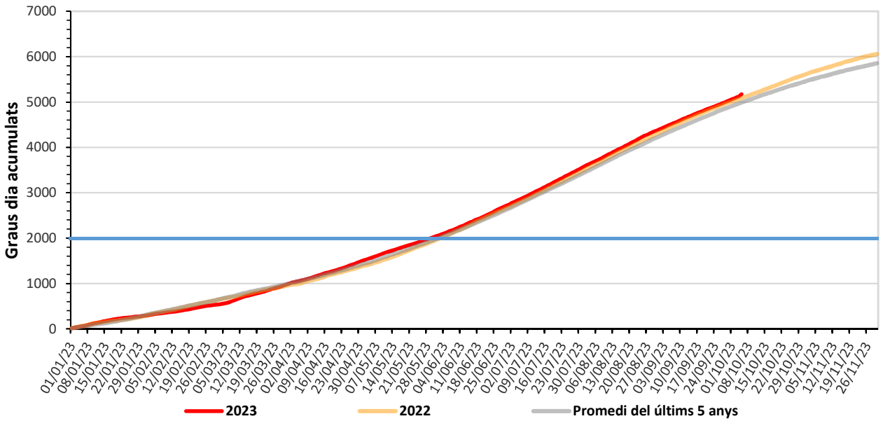
Grados dia acumulados València Interior
